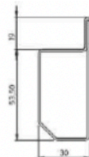
Coupe du longeron
