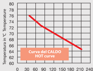
PROVA DI EFFICACIA DI ISOLAMENTO TERMICO EFFETTUATO CON PRODOTTI CALDI E FREDDI INSULATING TEST MADE ON COLD AND HOT SAMPLES
