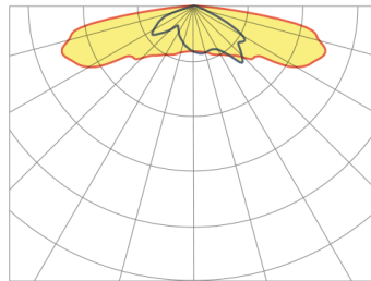
ASYMETRIQUE (A4)
