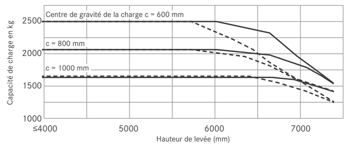
RX 60-25/600 avec mât triplex
