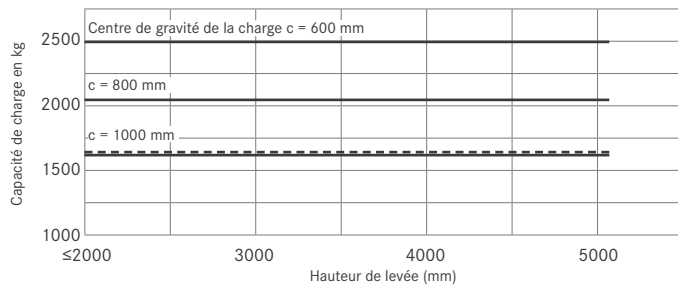
RX 60-25L/600 avec mât télescopique/HiLo
