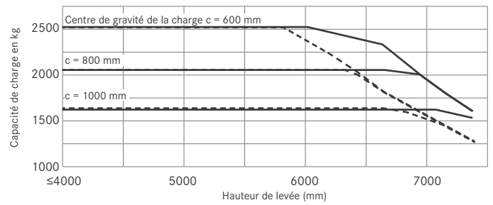
RX 60-25L/600 avec mât triplex
