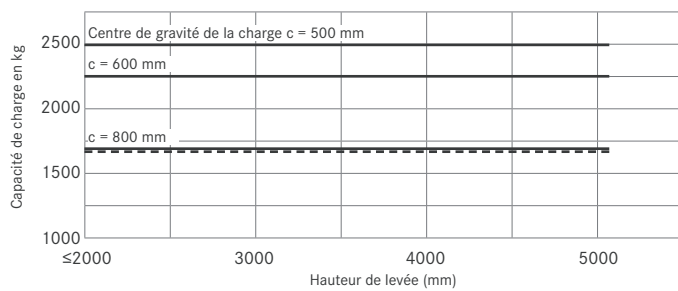
RX 60-25 avec mât télescopique/HiLo
