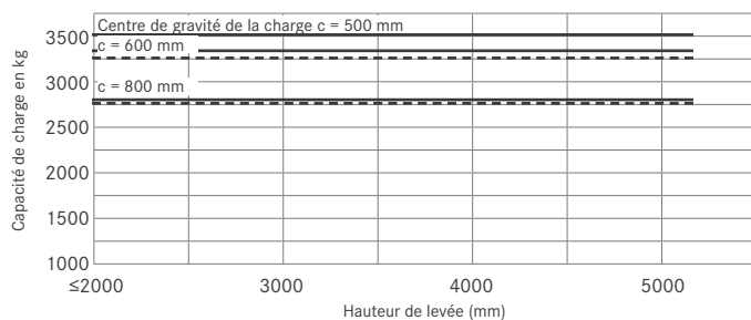
RX 60-35L avec mât télescopique/HiLo
