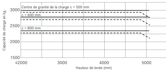
RX 60-30L avec mât télescopique/HiLo
