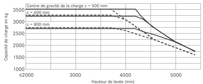
RX 60-35L avec mât triplex
