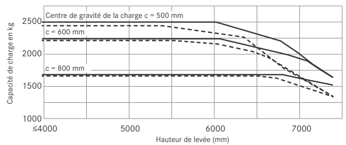
RX 60-25 avec mât triplex
