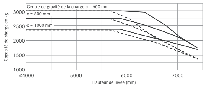
RX 60-30L/600 avec mât triplex
