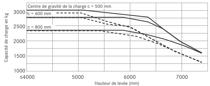
RX 60-30L avec mât triplex
