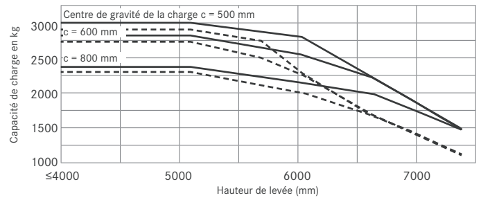
RX 60-30 avec mât triplex
