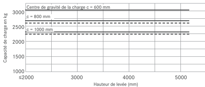
RX 60-30L/600 avec mât télescopique/HiLo
