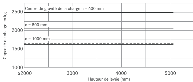
RX 60-25/600 avec mât télescopique/HiLo
