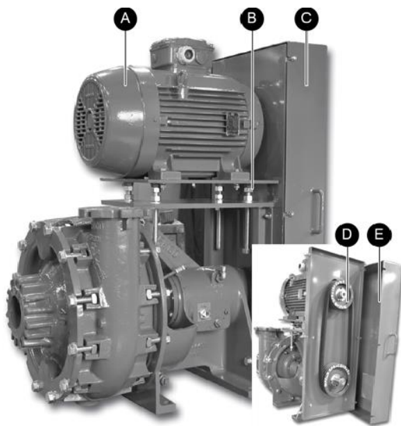
Figure 1 Vue générale avant et arrière d'un ensemble électropompe sur châssis de type MT.
