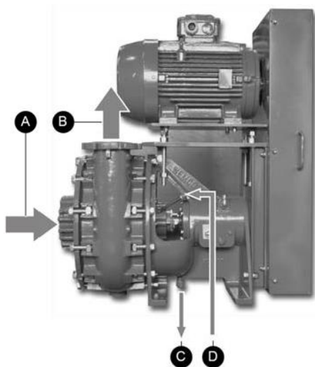
Figure 10 Plan général des tuyauteries périphériques à la pompe.
