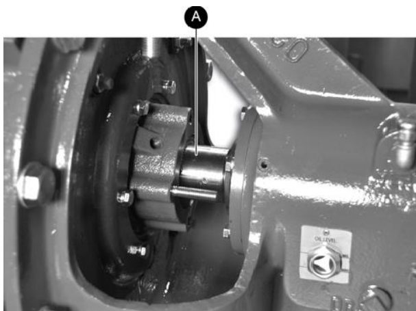
Figure 49 Le presse-étoupe ôté, l'arbre de pompe (A) est visible.
