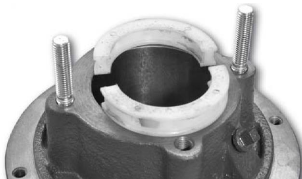
Figure 40 Mise en place de la lanterne d'arrosage en second
