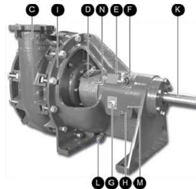
Figure 3 Vue générale arrière de la pompe.
