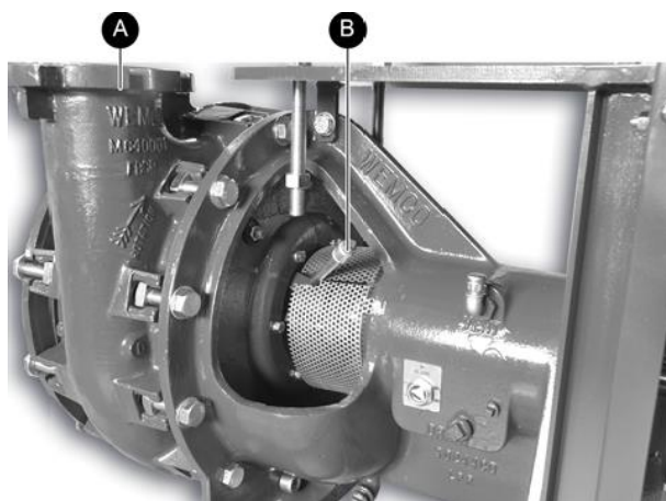
Figure 45 L'orifice u tube d'alimentation en eau des tresses (B) doit toujours se situer côté refoulement (A),
