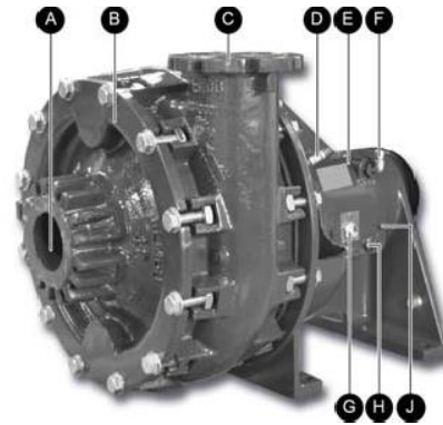
Figure 2 Vue générale avant de la pompe.
