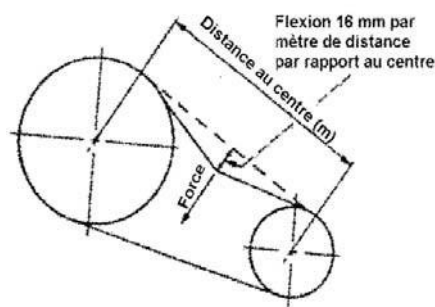
Figure 26 Principe de l'écart en fonction d'une force
