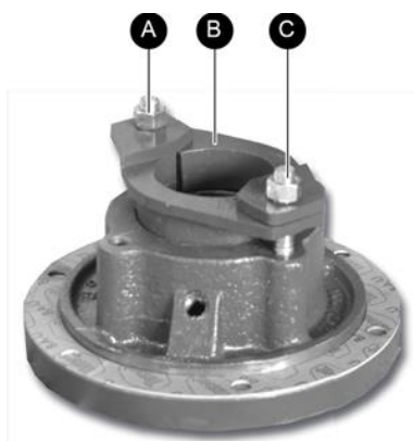
Figure 37 Dépose les deux écrous du fouloir de presse-étoupe.
