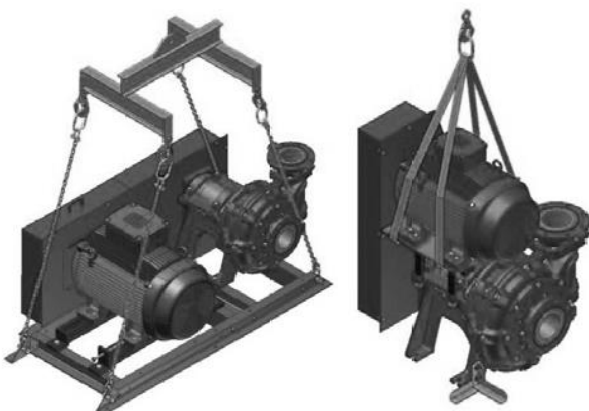
Figure 8 Levage d'une pompe sur châssis CL ou MT
