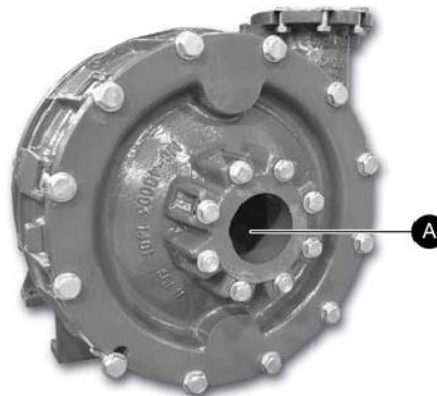
Figure 5 Vérification de l'absence d'éléments étrangers dans l'impulseur.
