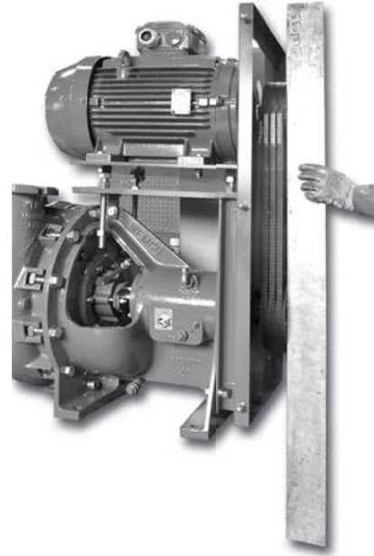
Figure 46 L'alignement correct des poulies s'effectue à l'aide d'un règle
