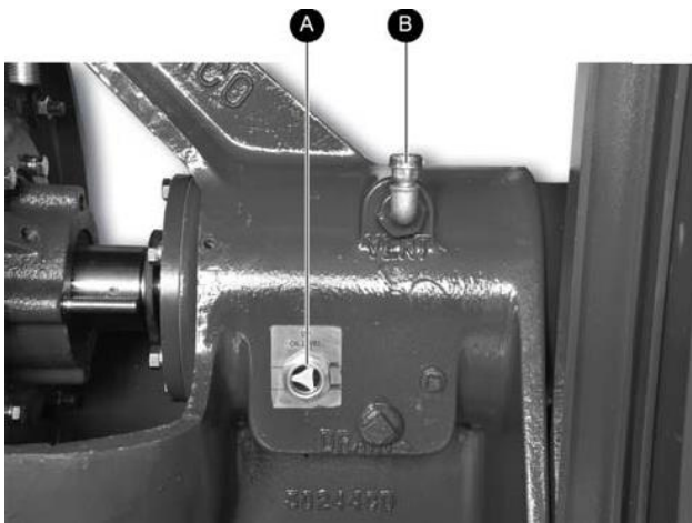
Figure 17 Le niveau d'huile (A) et le remplissage d'huile (B)
