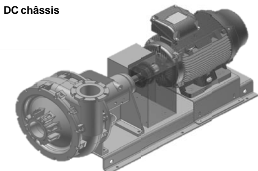
Figure 4 Différents châssis disponibles
