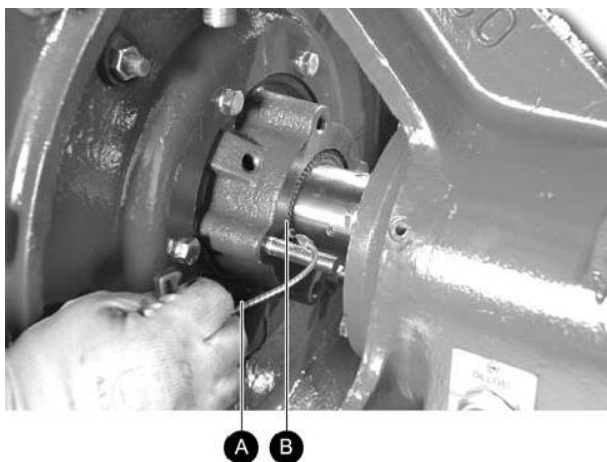
Figure 50 L'extracteur à tire-bouchon permet d'extraire les 3 premières tresses, la lanterne et la 4 ème tresse du fond.
