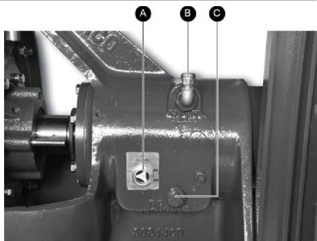
Figure 23 Localisation du niveau (A) et le remplissage d'huile (B).
