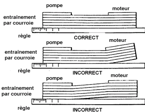
Figure 25 Principe d'alignement des courroies
