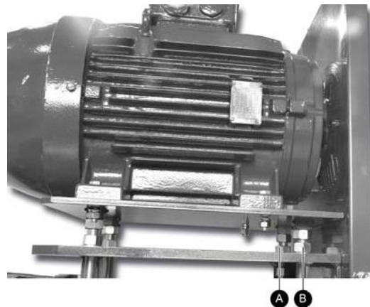
Figure 20 Les écrous du support moteur servent à tendre les courroies,
