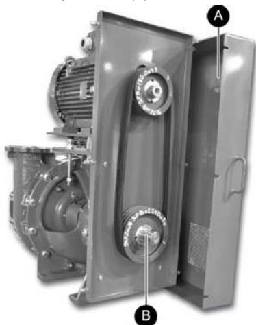
Figure 18 Dépose du carter de protection sur un ensemble pompe-moteur
