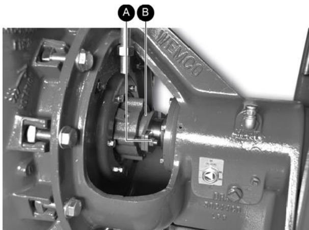
Figure 48 Les 2 écrous (A) du presse-étoupe (B).
