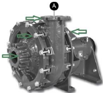
Figure 13 Localisation de la sortie (refoulement de la pompe). Position des boulons de serrage du corps et des brides
