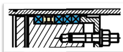
Figure 38 Empilage des tresses d'étanchéité et lanterne d'arrosage
