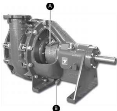
Figure 25 Localisation du raccord d'alimentation (A) et d'évacuation (B) en eau de l'étanchéité de la pompe.
