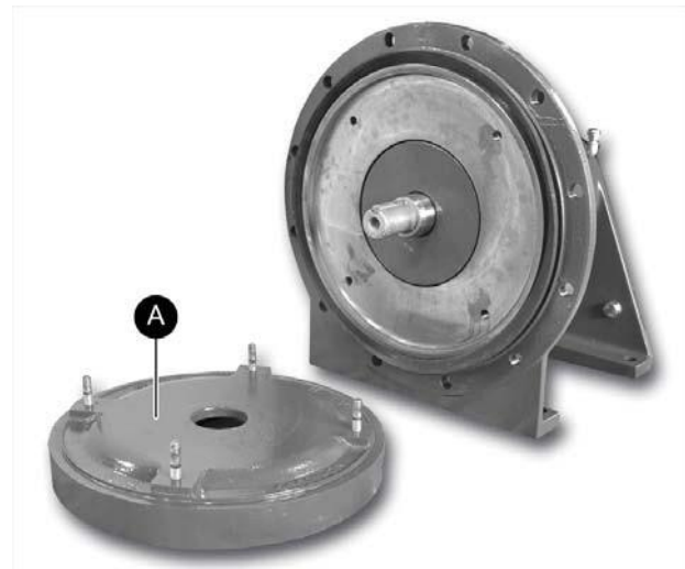
Figure 32 Dépose de la cuvette (A).
