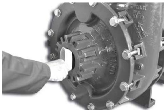
Figure 9 Cape plastique à retirer juste avant la connexion de la bride.
