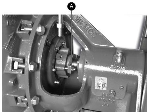
Figure 46 Les écrous de réglage du fouloir de presse-étoupe.
