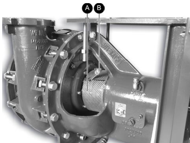
Figure 47 La grille de protection (A) et déposer le tube d'arrosage de tresses (B).
