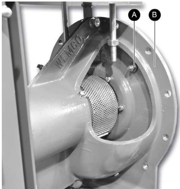
Figure 31 Les 4 écrous (A), rondelles bombées et rondelles caoutchouc en partie arrière de la boîte support (B).
