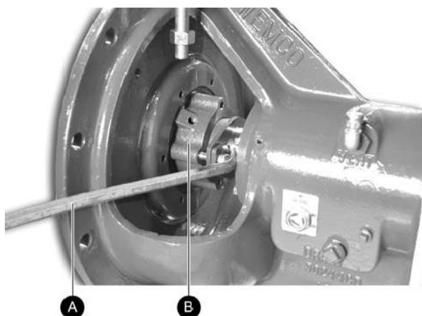
Figure 35 Le boîtier presse-étoupe (B) est poussée vers l'avant à l'aide d'un levier (A).
