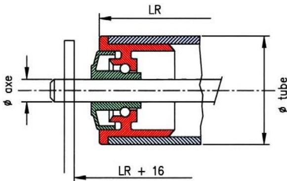
Rouleaux libres avec roulements de manutention
