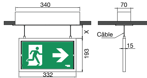
Encastré Béton - EB
