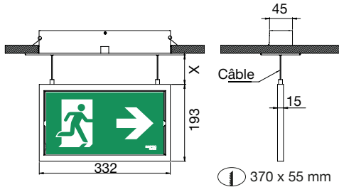
Faux plafond - EM
