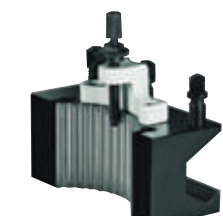
Vue arrière du porte-outil type H
