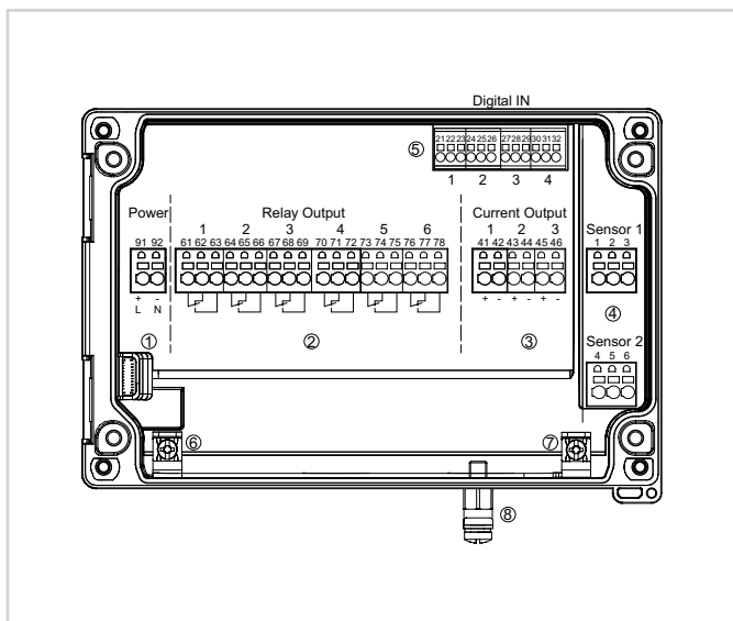
Schéma de raccordement VEGAMET 862
