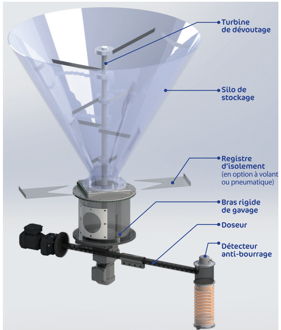
Exemple d'implantation :
