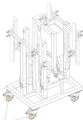
Chariot de transport sur roues
