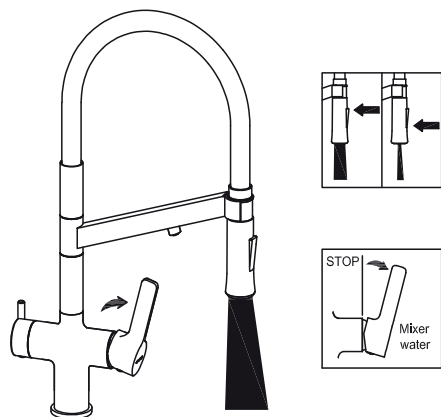
Salida de agua mezclada / Mixed water outlet
