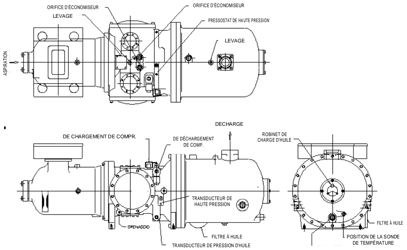
Fig. 17 - Installation des dispositifs de contrôle pour le compresseur Fr 3200
