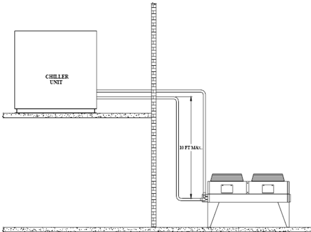
Fig. 8 - Condenseur positionné en dessous de l'unité de refroidisseur
