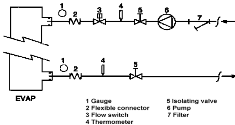
Fig. 4 - Raccordement des tuyaux d'eau pour les échangeurs de récupération de chaleur
