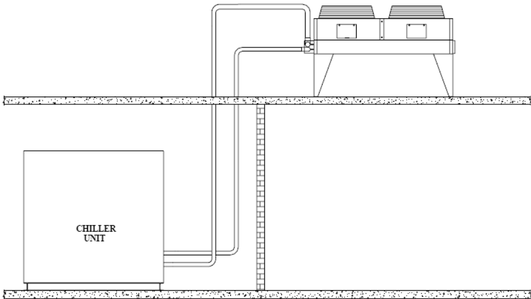
Fig. 7 - Condenseur positionné au-dessus de l'unité de refroidisseur
