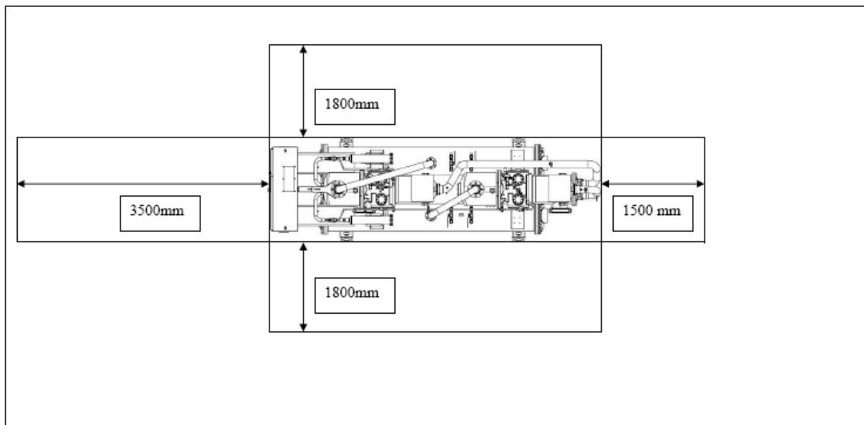
Fig. 2 - Exigences de dégagement minimales pour l'entretien de la machine
