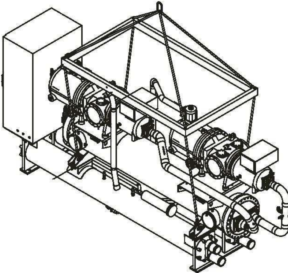
Fig. 1 - Levage de l'unité
