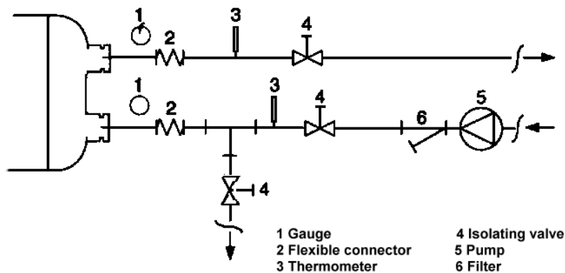
Fig. 3 - Raccordement des tuyaux d'eau de l'évaporateur
