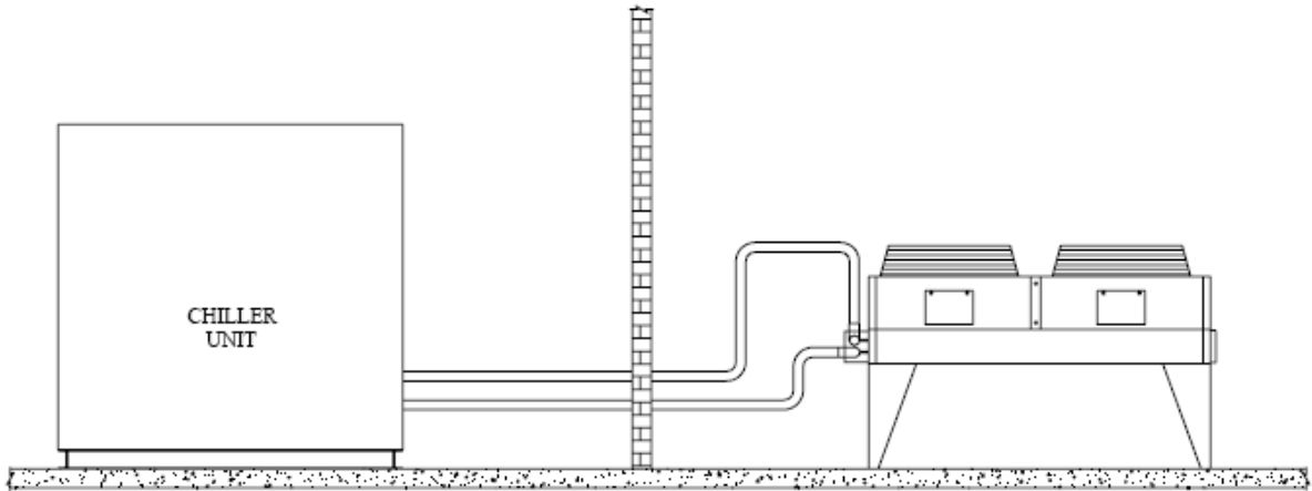
Fig. 6 - Condenseur positionné sans différence d'élévation
