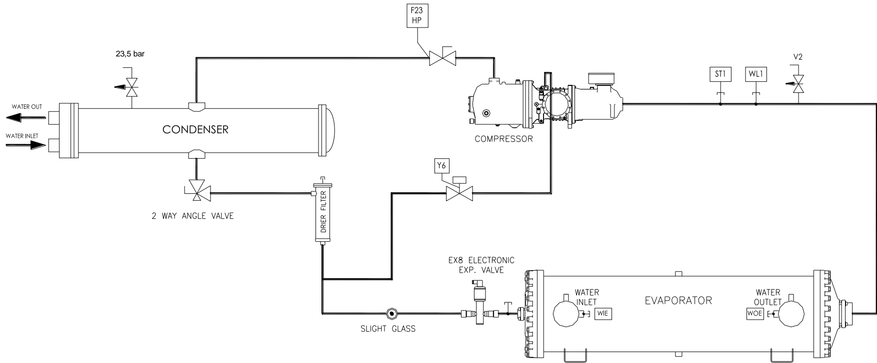
Fig. 10 - Cycle de réfrigération EWWD G-SS / EWWD G-XS
