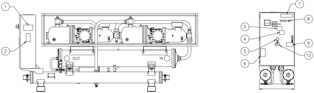
Unité à deux compresseurs
