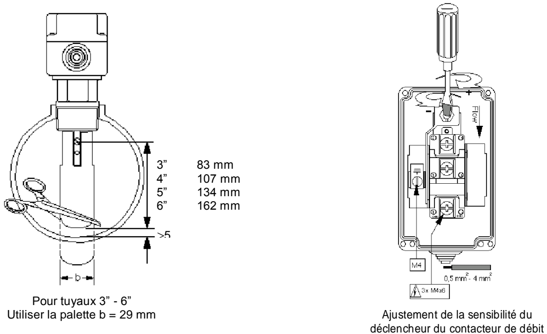
Fig. 5 - Ajustement du contacteur de débit de sécurité
