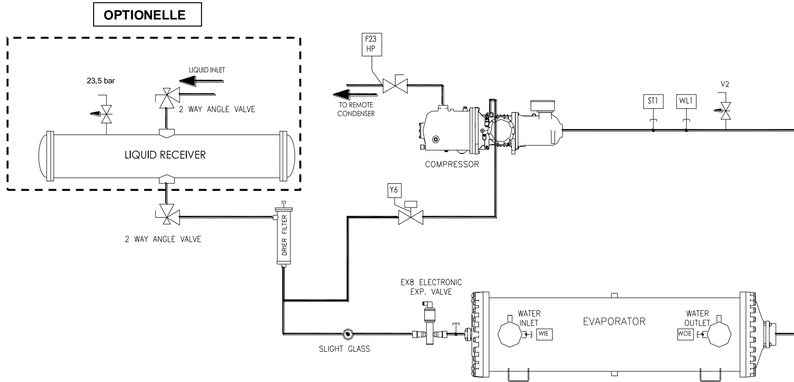
Fig. 12 - Cycle de réfrigération EWLD G-SS
