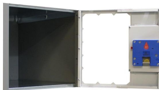
Détail de la Porte transparente et de la serrure à clé prisonnière - monayeur à 2€
