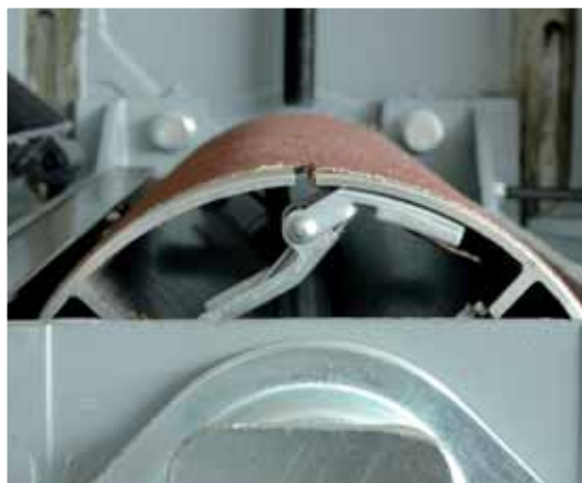
Cylindre en aluminium avec gâchette de blocage rapide
