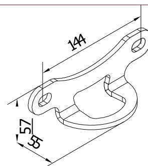
Platine d'extrémité
