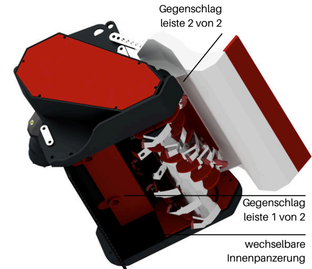
Spezial Randwerkzeug
