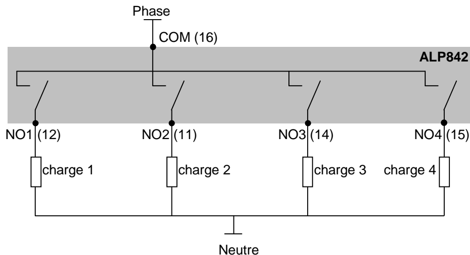
△ Câblage de 4 charges (230Vac, 5A max) sur les 4 relais
