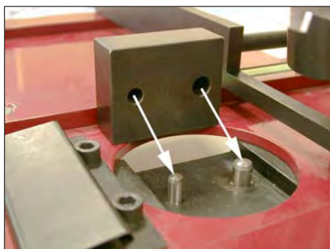
Mise en place de l'Enclume et de l'Attache. Les attaches n'ont qu'une position possible sur l'enclume.
