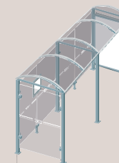
Lérins - Longueur 5000 Une vitrine 2000 + un bardage latéral Réf. 529339
