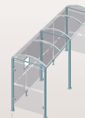
Noirmoutier - Longueur 5000 Deux bardage latéraux Réf. 529319
