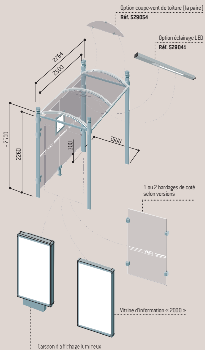
Modèle présenté : Adour-RAL 6005 - Pommeaux Agora - Réf. 529312
