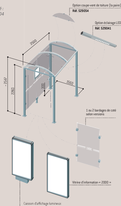
Modèle présenté : Lérins - RAL 8017 - Réf. 529338
