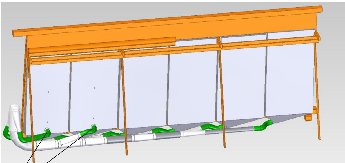
Vue arrière du système de captage GIRPAN ® installé sur la scie à panneaux
