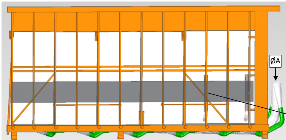
Scie à panneaux équipée du système de captage GIRPAN ® (Ø A : Aspiration secondaire)
