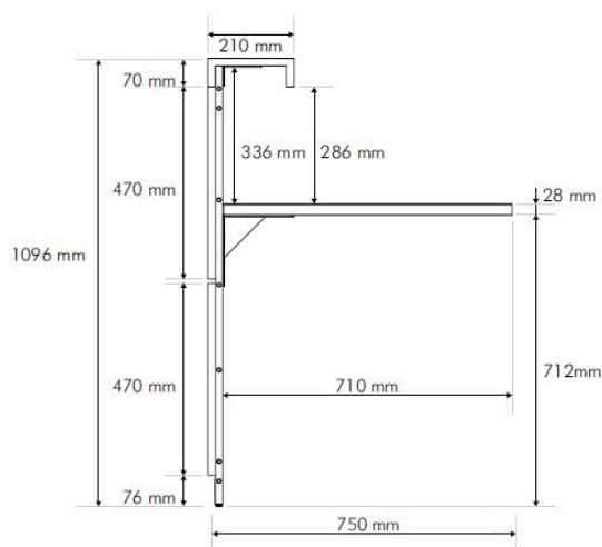
Module haut
