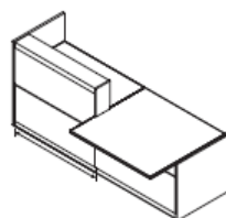
Banque droite PMR L246 à 326 cm x P105 cm
