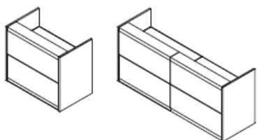
Banque droite haute, parois latérales 1 module : L120 à 200 cm x P75 cm ou 2 modules : L246 à 406 cm
