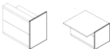
Paroi latérale ou intermédiaire H109 ou 74 x L2,8 x P75 cm
