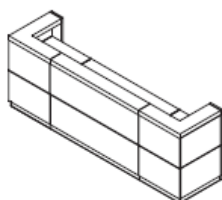
Banque droite haute, angles 90° L270 à 350 cm x P78 cm
