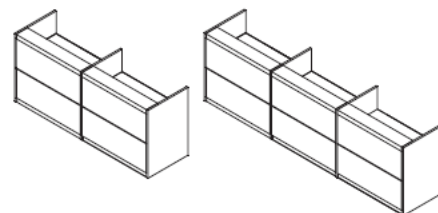
Banque droite haute, parois latérales avec parois intermédiaires 2 modules : L249 à 409 cm x P75 cm ou 3 modules : L372 à 492 cm
