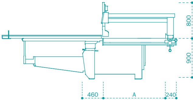
T60C | Vue de profil
