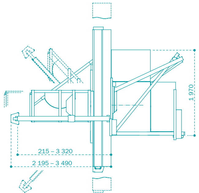
T60C | Vue du dessus
