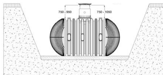
Maxi rehausse télescopique + Rehausse télescopique avec couverture en fonte
