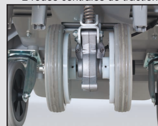
2 roues centrales de traction
