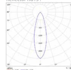
Reflector RG15 :
