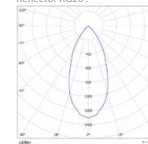
Reflector RG20 :
