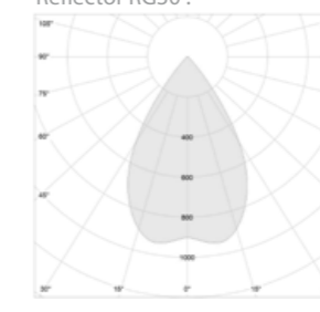
Reflector RG30 :
