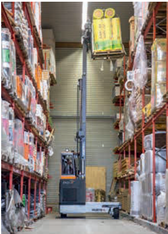
Chariot quadri-directionnel avec un moteur diesel au rendement énergétique optimisé Carrello elevatore a quattro vie con motore diesel ad alta efficienza
