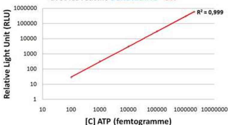
Calibration ATP du luminomètre Kikkoman C-110 avec les réactifs DENDRIDIAG® SW
