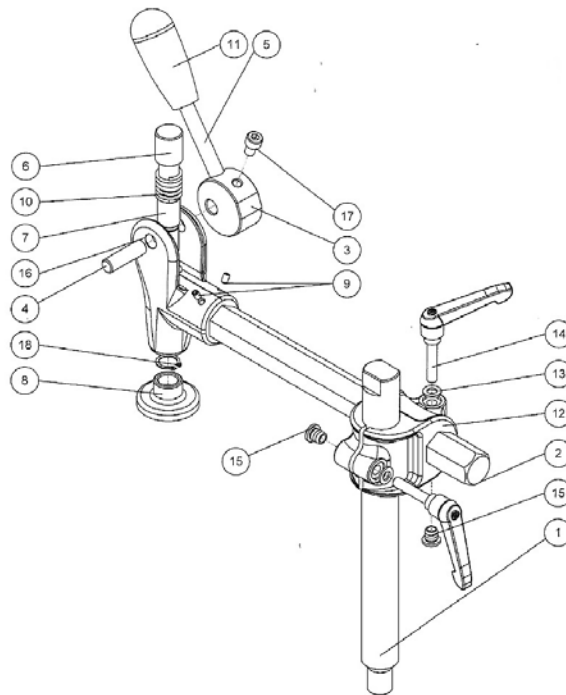
Abb. / Fig. 20: Ersatzteilzeichnung 20 / Spare parts drawing 20
