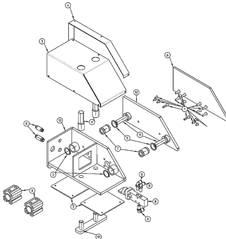
Abb. / Fig. 21: Ersatzteilzeichnung 21 / Spare parts drawing 21
