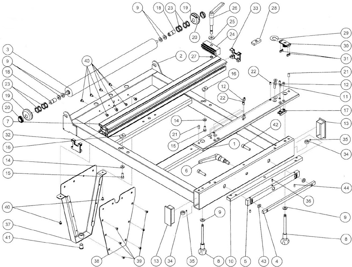
Abb. / Fig. 17: Ersatzteilzeichnung 17 / Spare parts drawing 17
