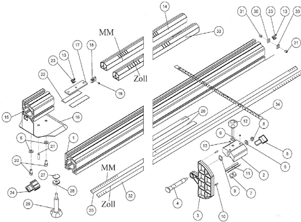
Abb. / Fig. 18: Ersatzteilzeichnung 18 / Spare parts drawing 18
