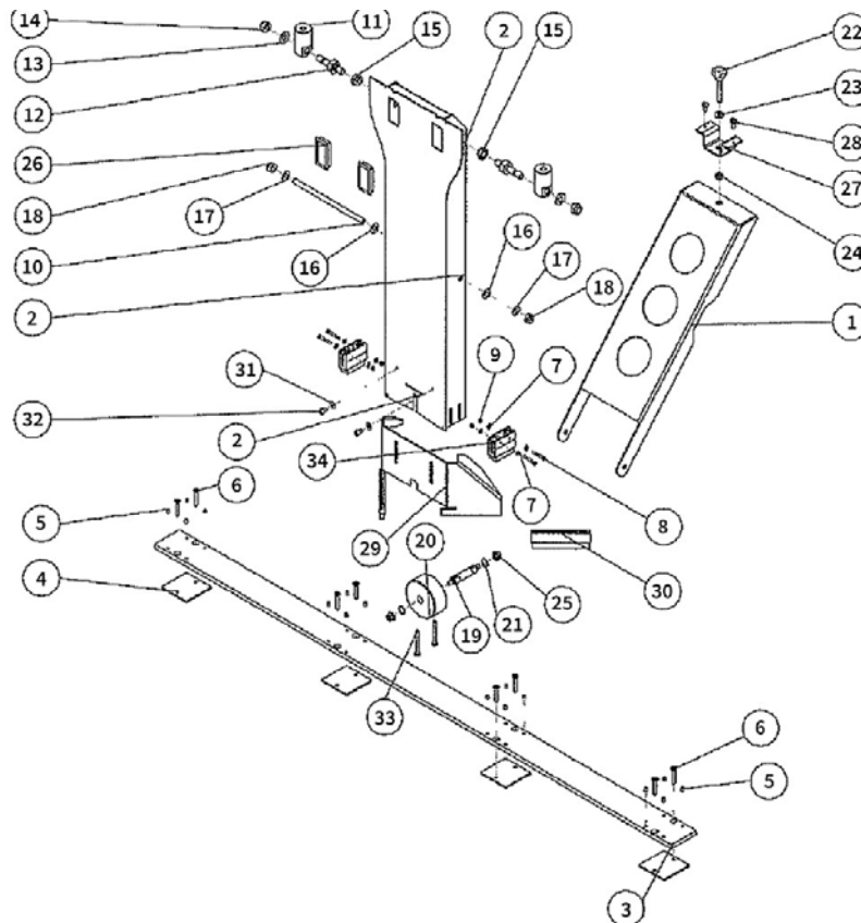
Abb. / Fig. 19: Ersatzteilzeichnung 19 / Spare parts drawing 19
