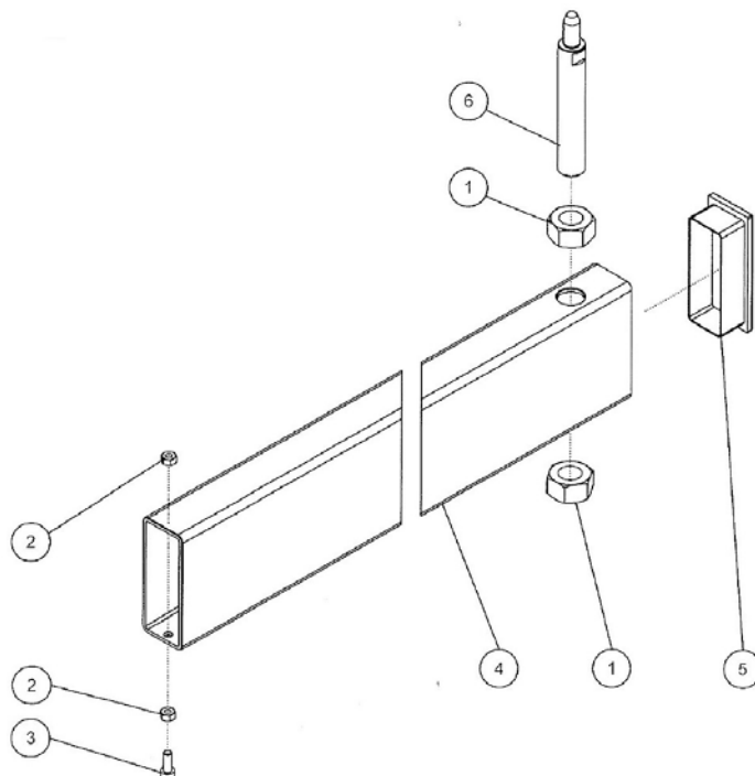
Abb. / Fig. 16: Ersatzteilzeichnung 16 / Spare parts drawing 16
