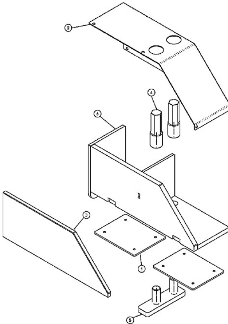
Abb. / Fig. 22: Ersatzteilzeichnung 22 / Spare parts drawing 22
