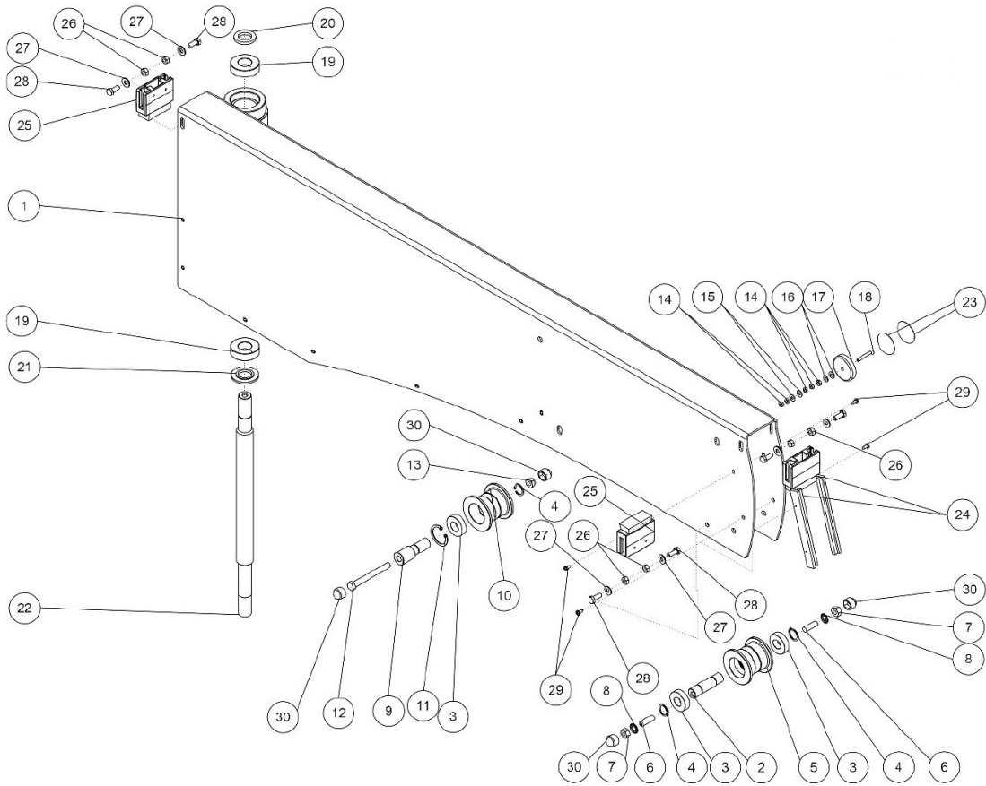
Abb. / Fig. 15: Ersatzteilzeichnung 15 / Spare parts drawing 15
