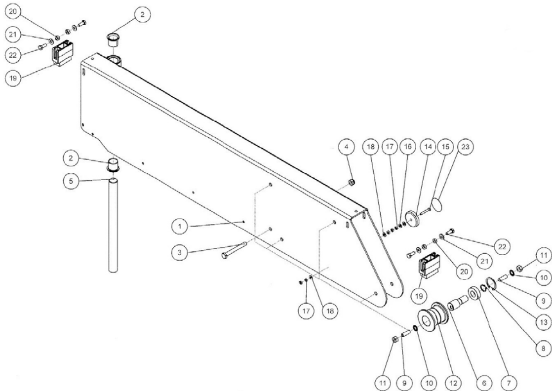
Abb. / Fig. 14: Ersatzteilzeichnung 14 / Spare parts drawing 14
