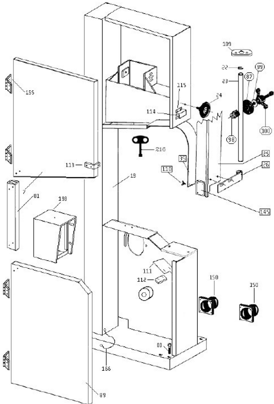
Abb. / Fig. 2: Ersatzteilzeichnung 2 / Spare parts drawing 2
