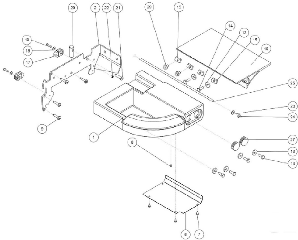
Abb. / Fig. 13: Ersatzteilzeichnung 13 / Spare parts drawing 13
