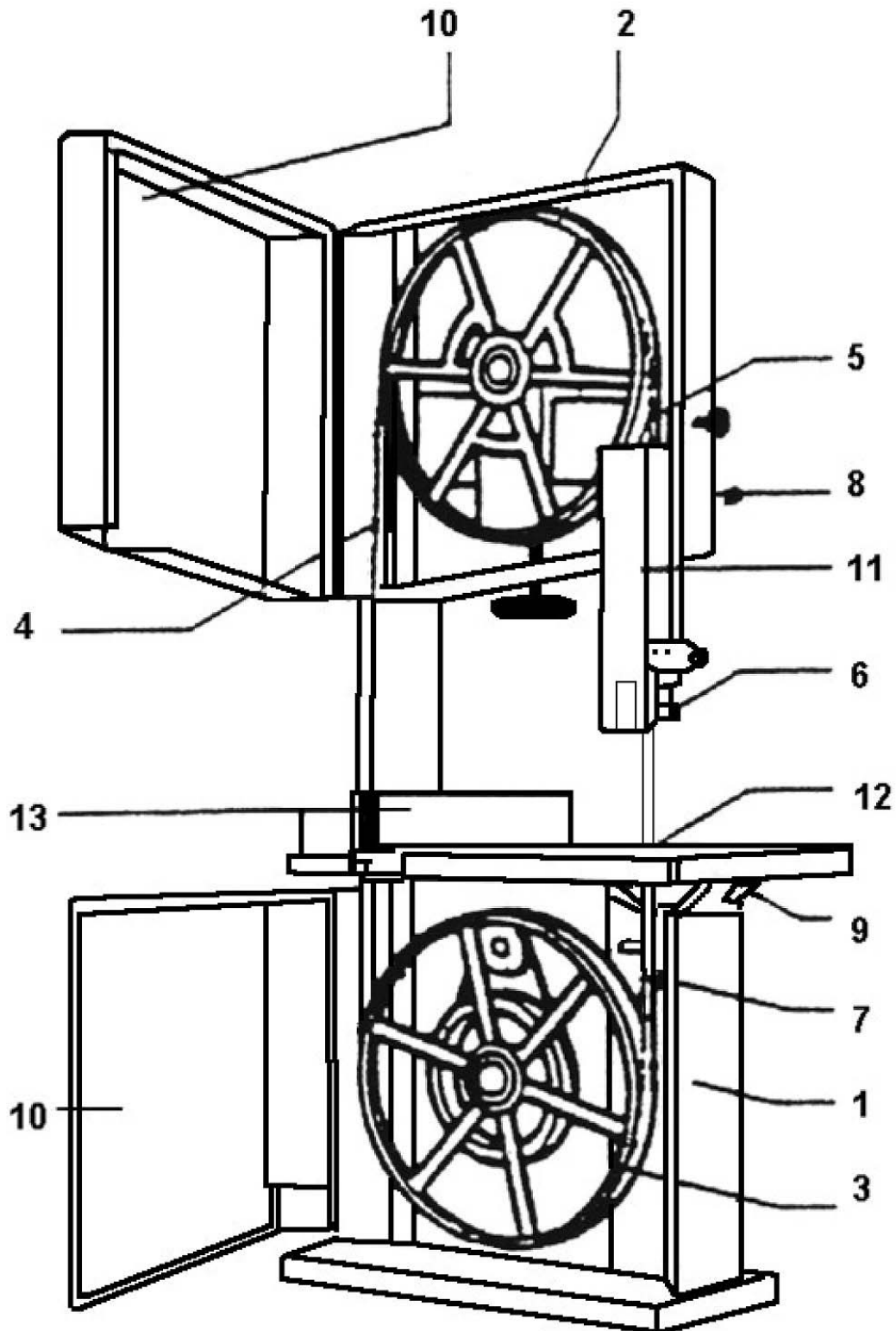
Abb. / Fig. 1: Ersatzteilzeichnung 1 / Spare parts drawing 1
