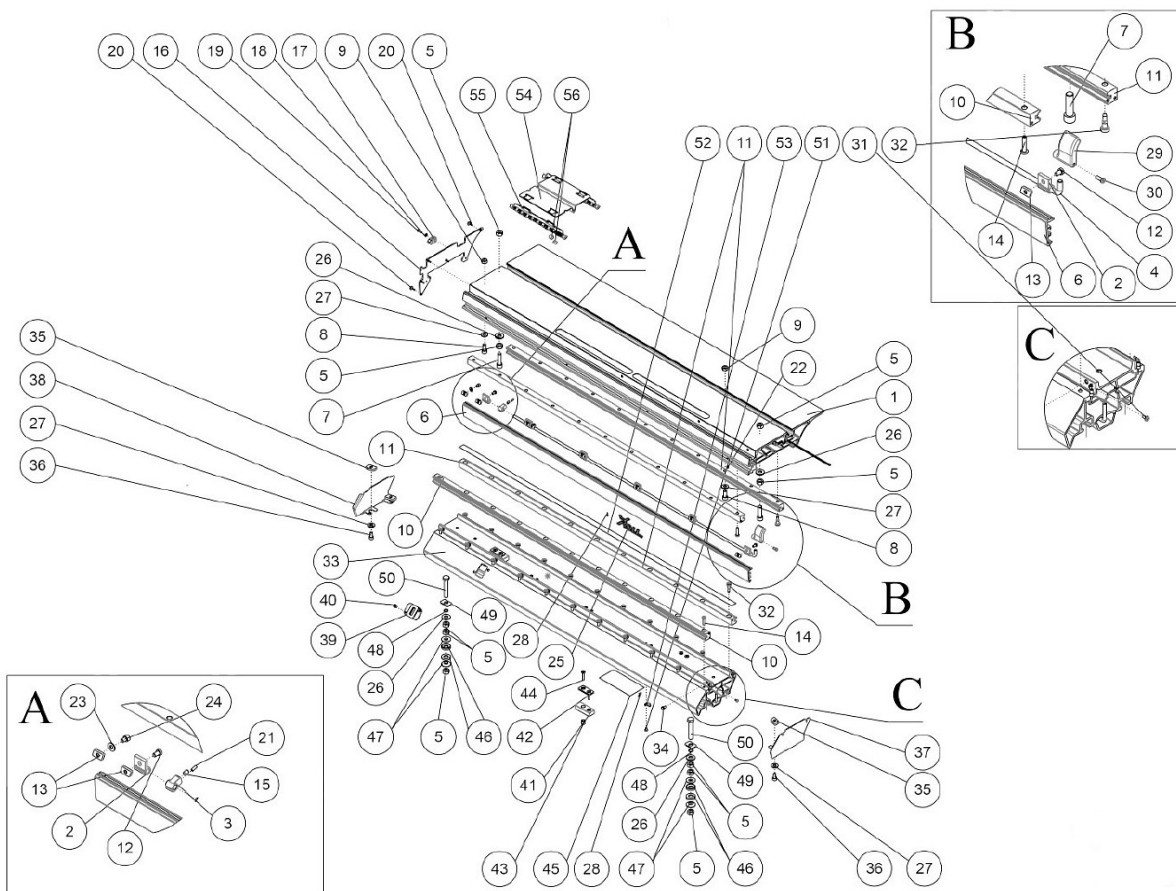
Abb. / Fig. 12: Ersatzteilzeichnung 12 / Spare parts drawing 12
