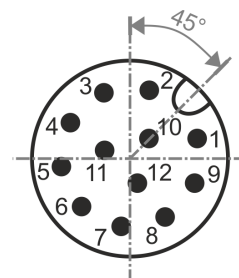
Vue sur la caméra (vue arrière)
