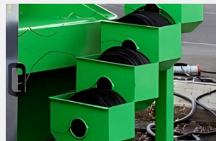
Supports de fil de 25 kg de série
