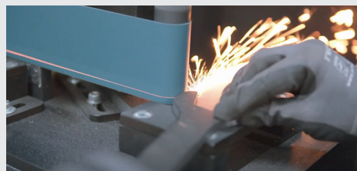
FIG: STATION DE PONÇAGE 1
