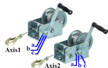
Fig.2b (PRTRM2000)
