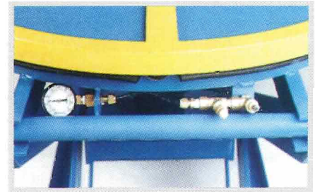
Le positionnement des manomètre et valve de commande à une extrémité de la table assure protection et accessibilité aisée
