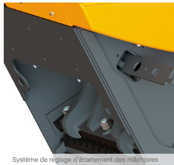
Bielle : pièce en acier coulé massif
