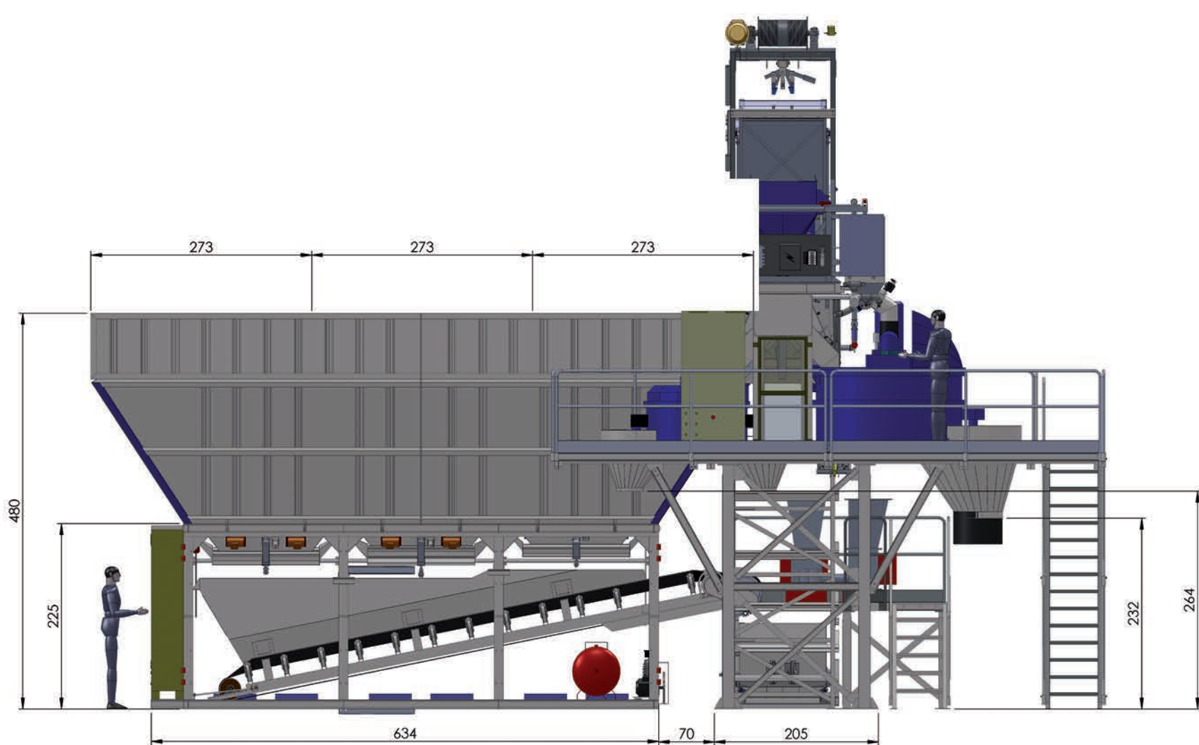
Vista Frontale
