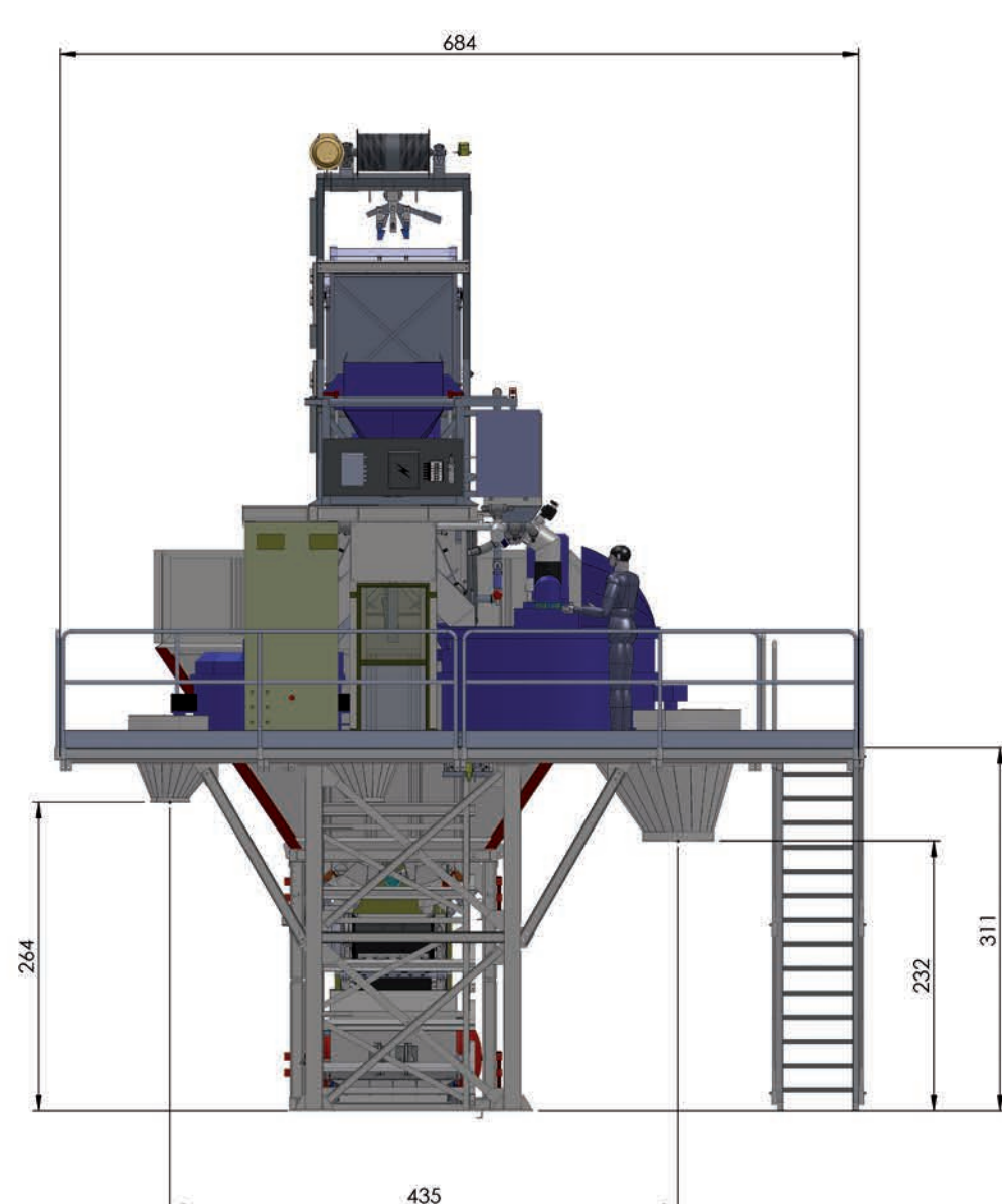
Vista laterale
