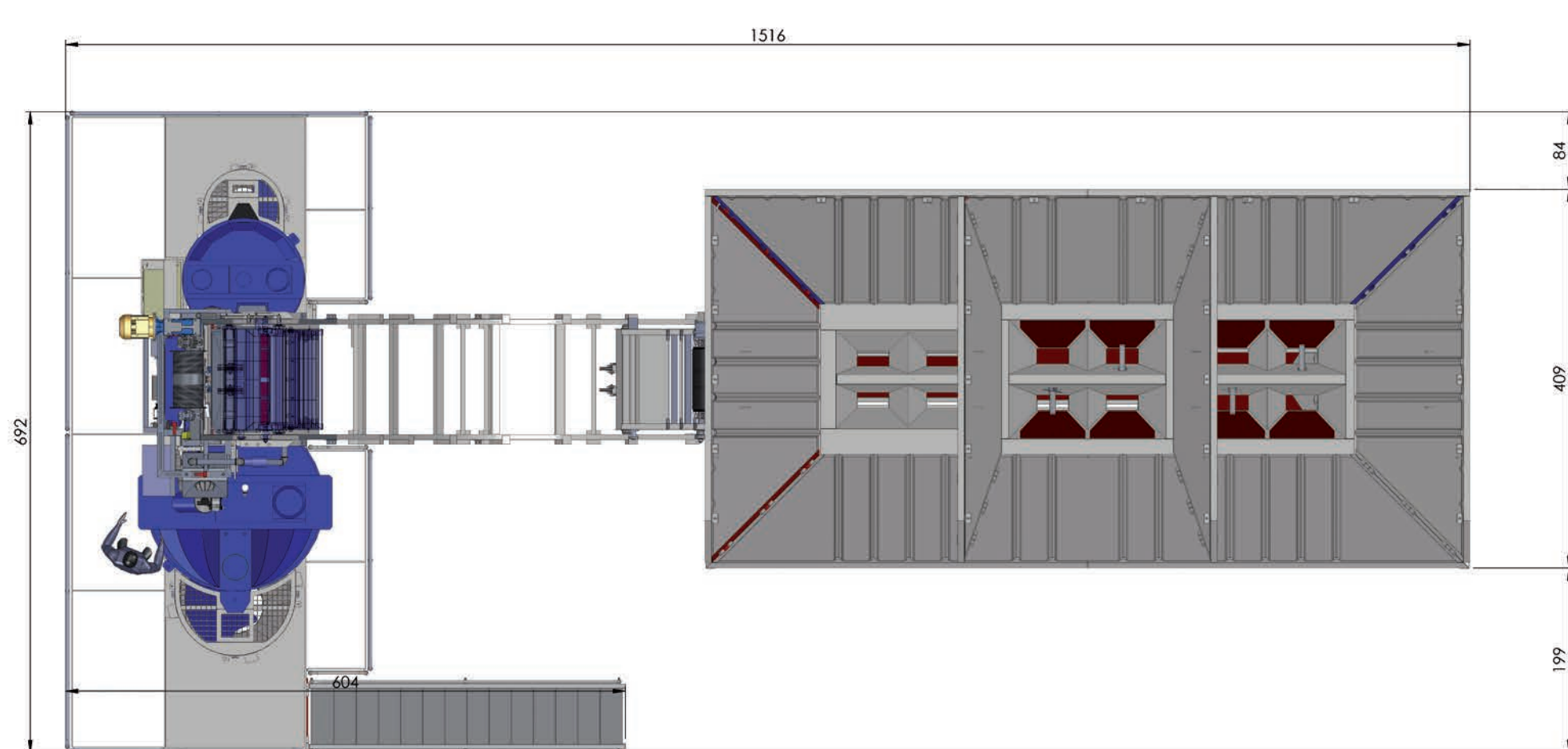
Vista dall'alto
