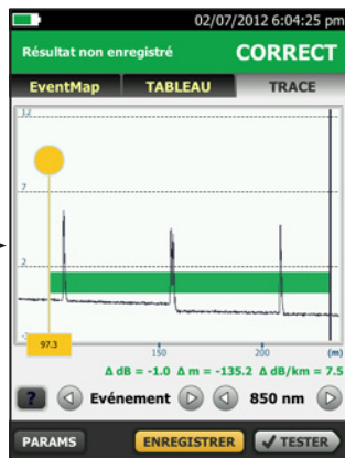
Résultat du test réflectométrique (zoom avant)
