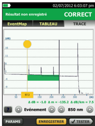
Résultat du test réflectométrique
