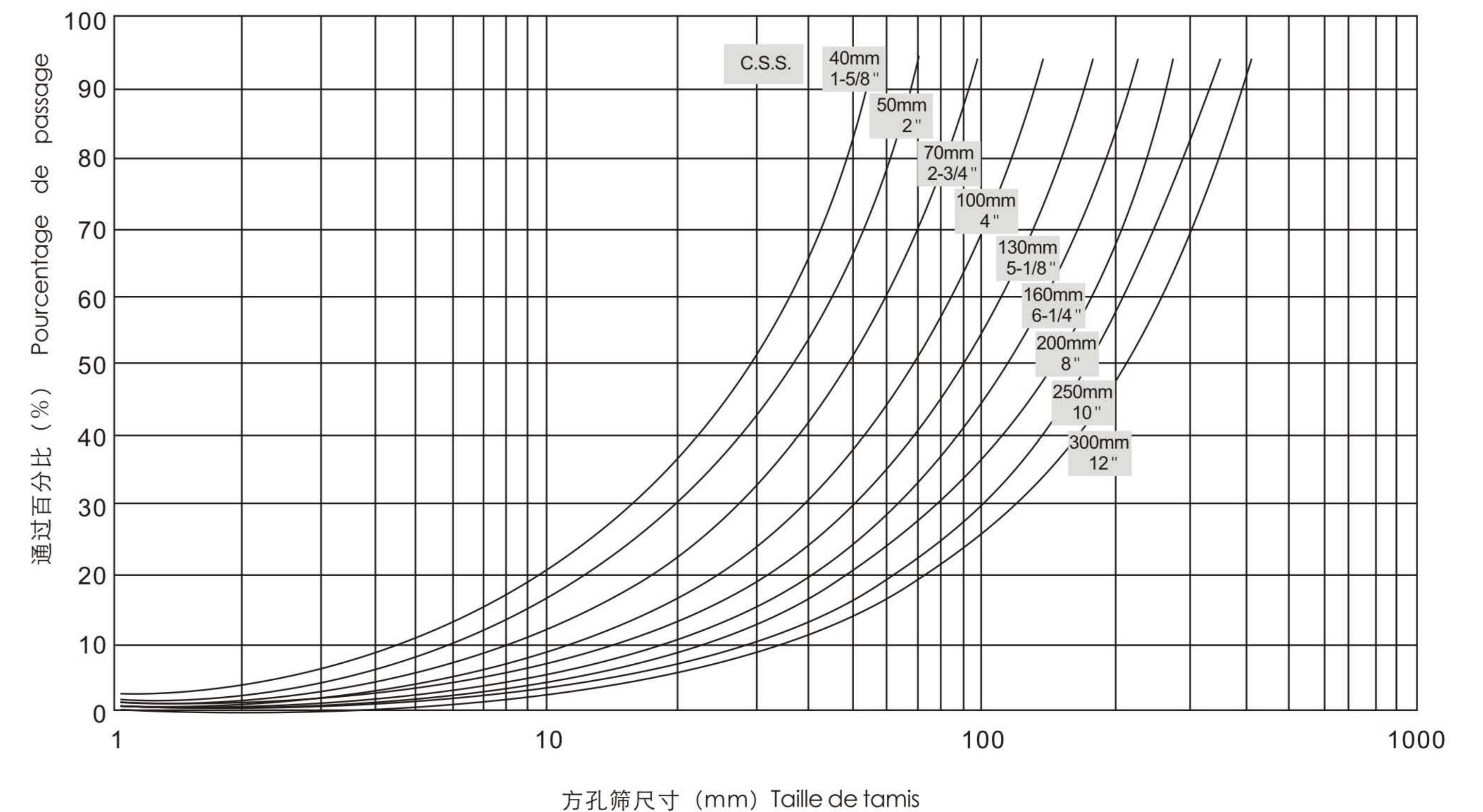
Courbes Granulométriques de Concasseur à Mâchoire
