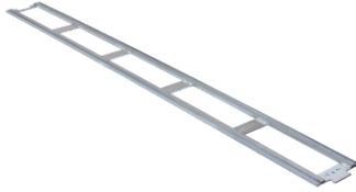
TRO-0475-13-00-00-0 Rail 1800 mm (70,9") avec rainures en "V" écartées de 152 mm (6")
