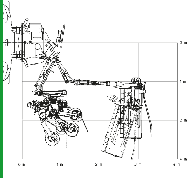
Diagramme de portées MLM 200
