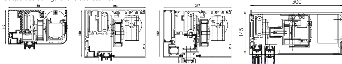
Coupe des configurations coulissantes
