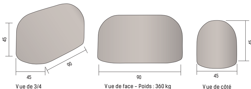
BORDURE ANTI-STATIONNEMENT ANTI-VOITURE BÉLIER
