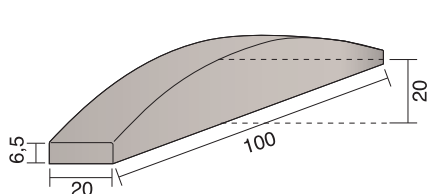
BORDURE ANTI-STATIONNEMENT NAUTILE
