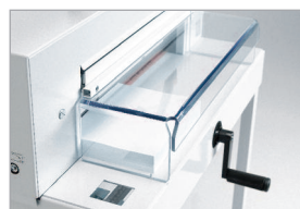
Carter de protection pivotant sur la table avant
