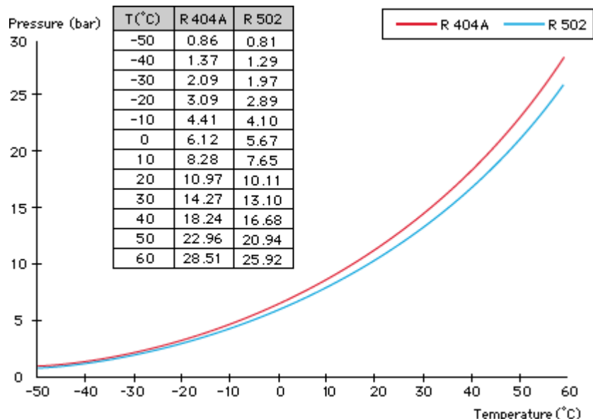
Graphique comparative température/pression du R-502 et R404A :
