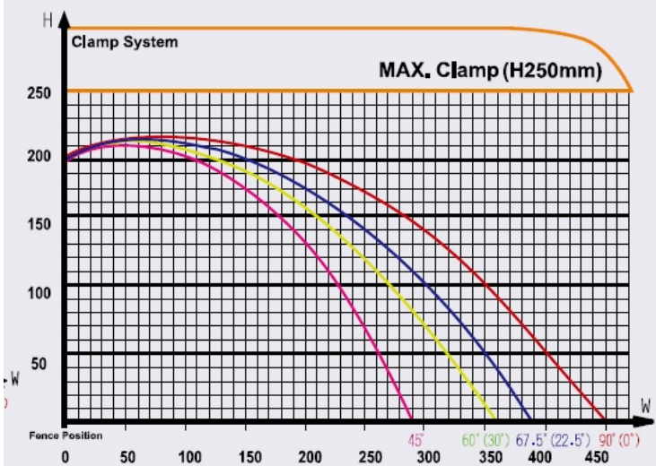
JIH-20 24 TYPE Diagramme de coupe
