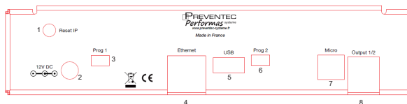
connectique de l'afficheur
