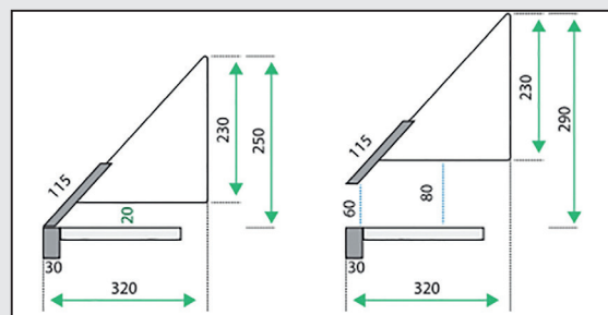
FIG : DIMENSIONS DES SEGMENTS E-AKB 3.020-1,2
