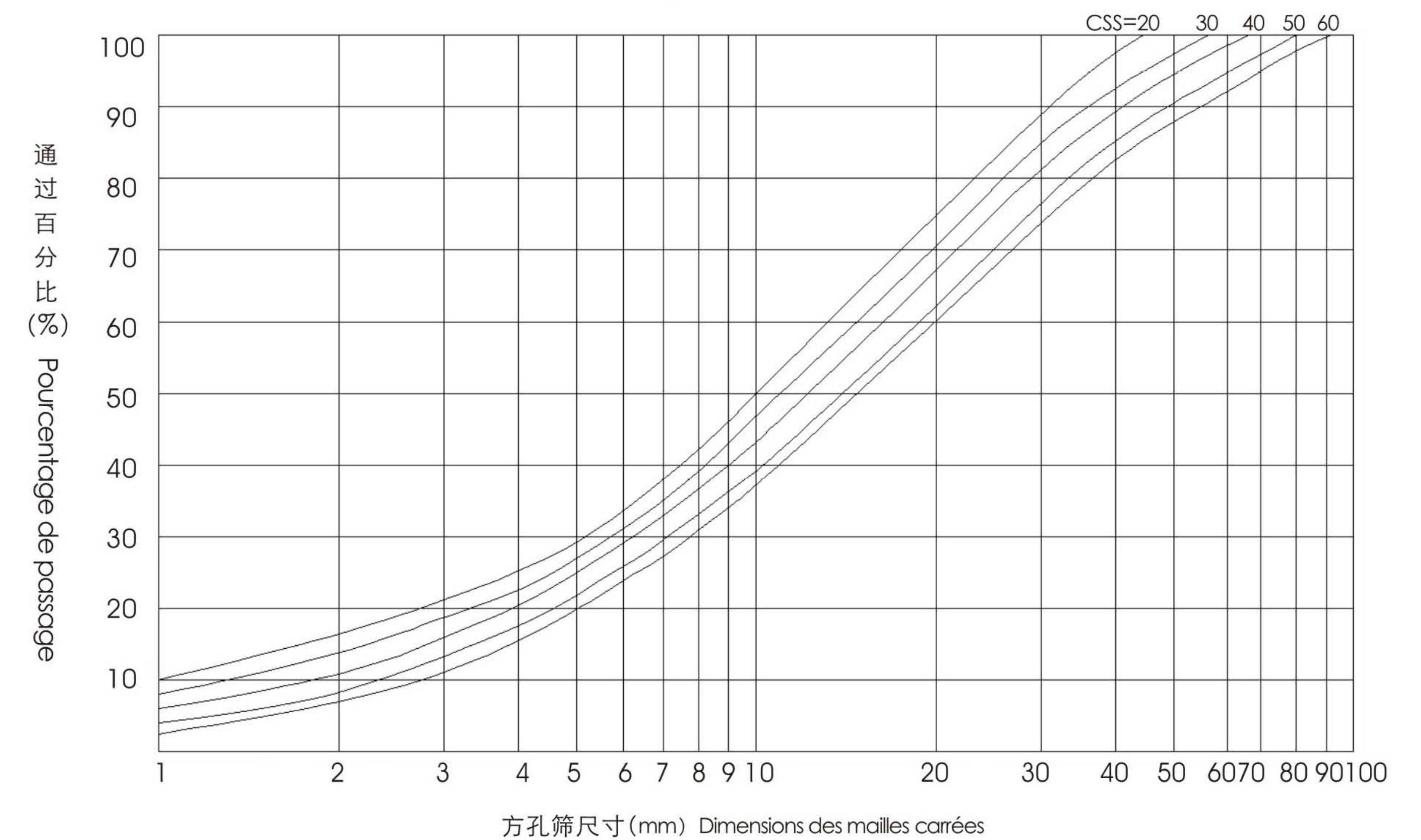
Courbes Granulométriques de Concasseur à Percussion
