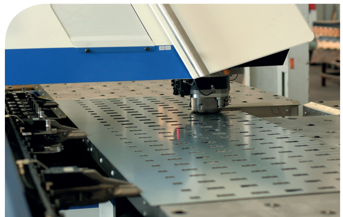
TopSolid'Sheetmetal propose des stratégies d'usinage pour chaque outil afin d'optimiser le parcours de la tête de poinçonnage sur la tôle
