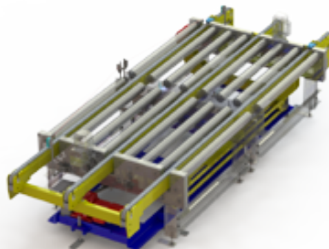
Transfert orthogonal avec convoyeur à chaînes
